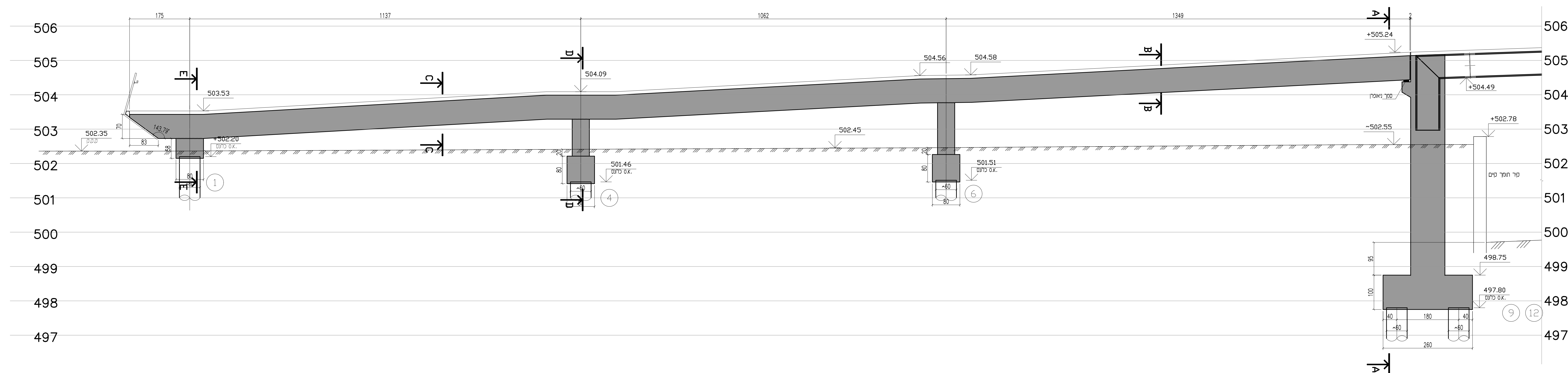
1:50 G-G חתר
