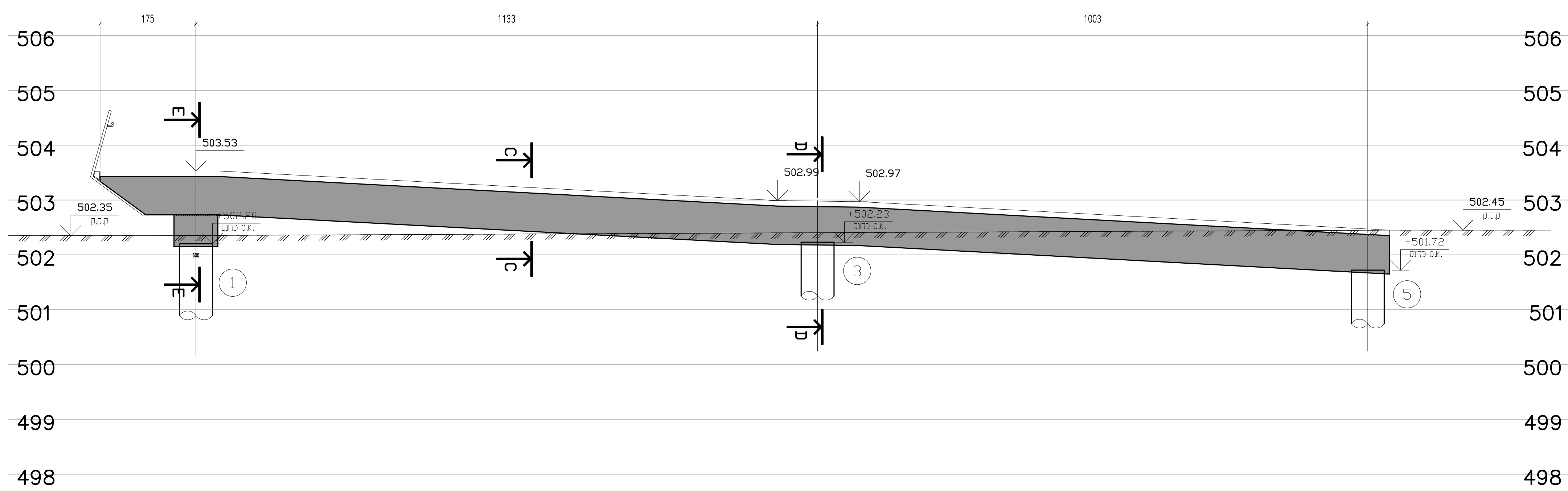
1:50 F-F חתך
