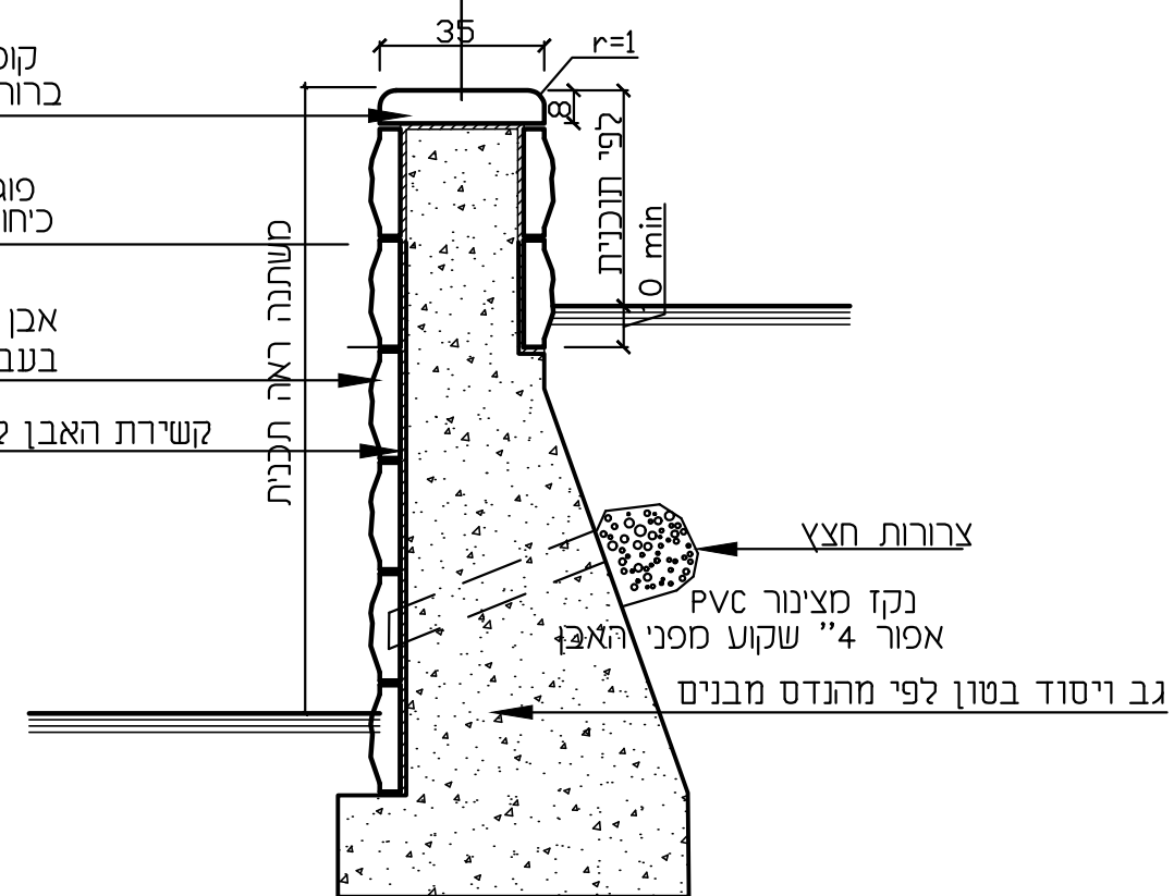
חתך 1:20
